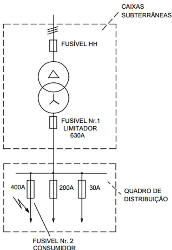
Figura 2 – Seletividade
